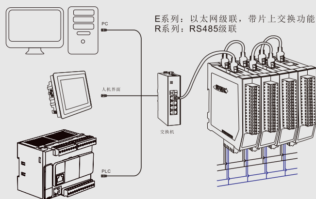
CK模块通过以太网接口级联组网连接示意图
